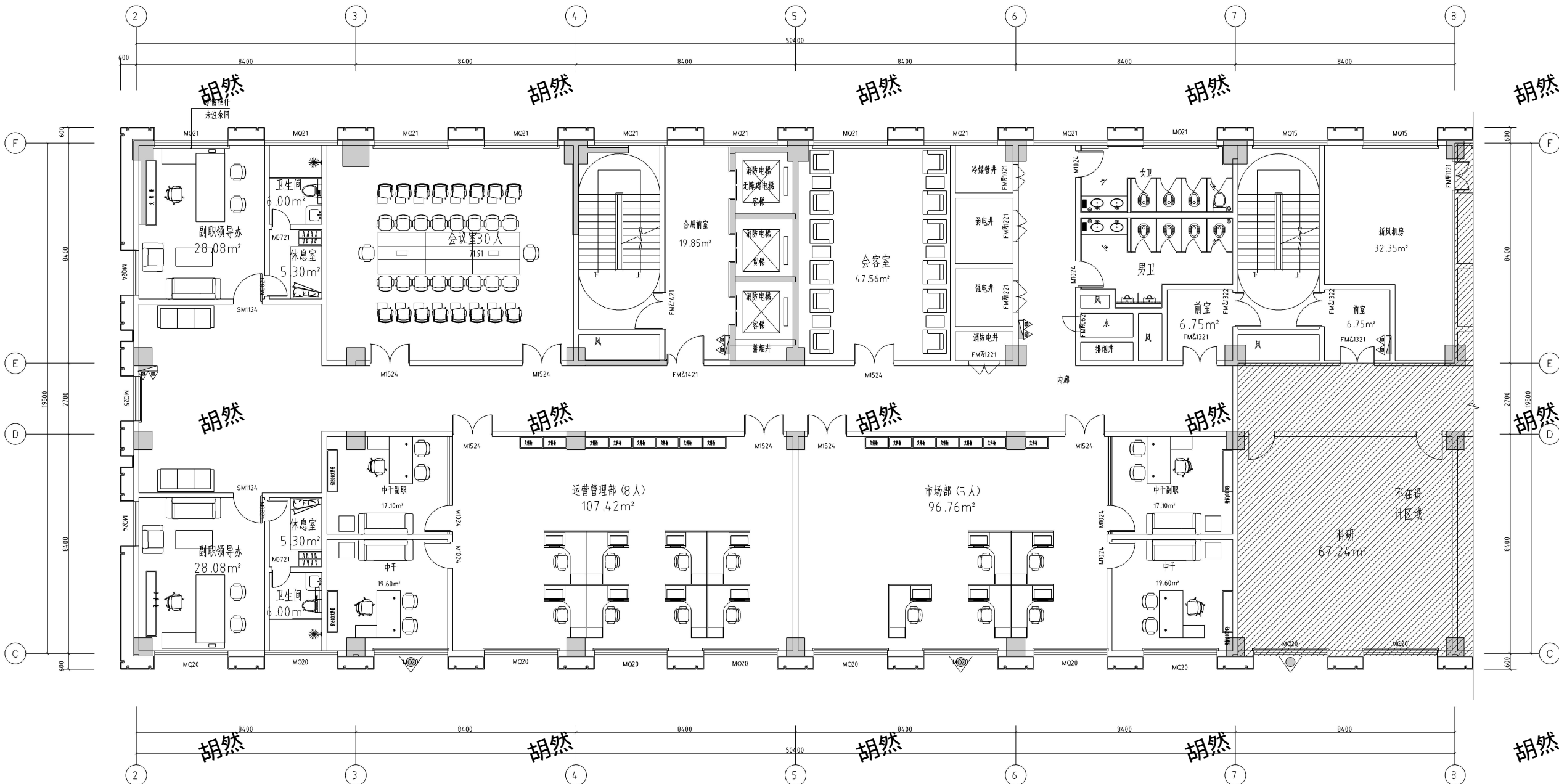
六层平面布置图 1:100
